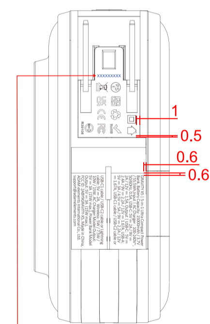
左視圖 (Cable拿出來後)
