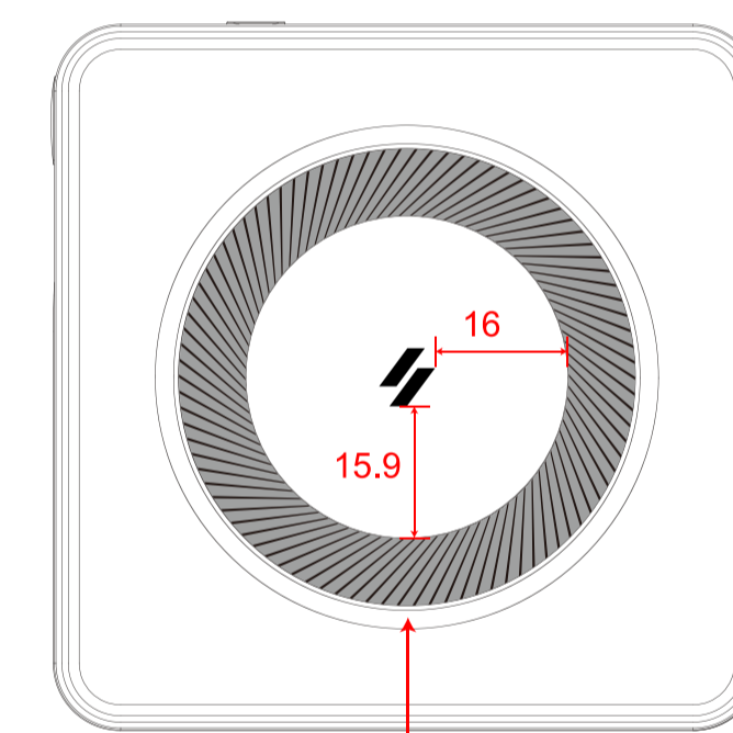
後視圖
