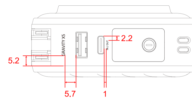
上視圖
