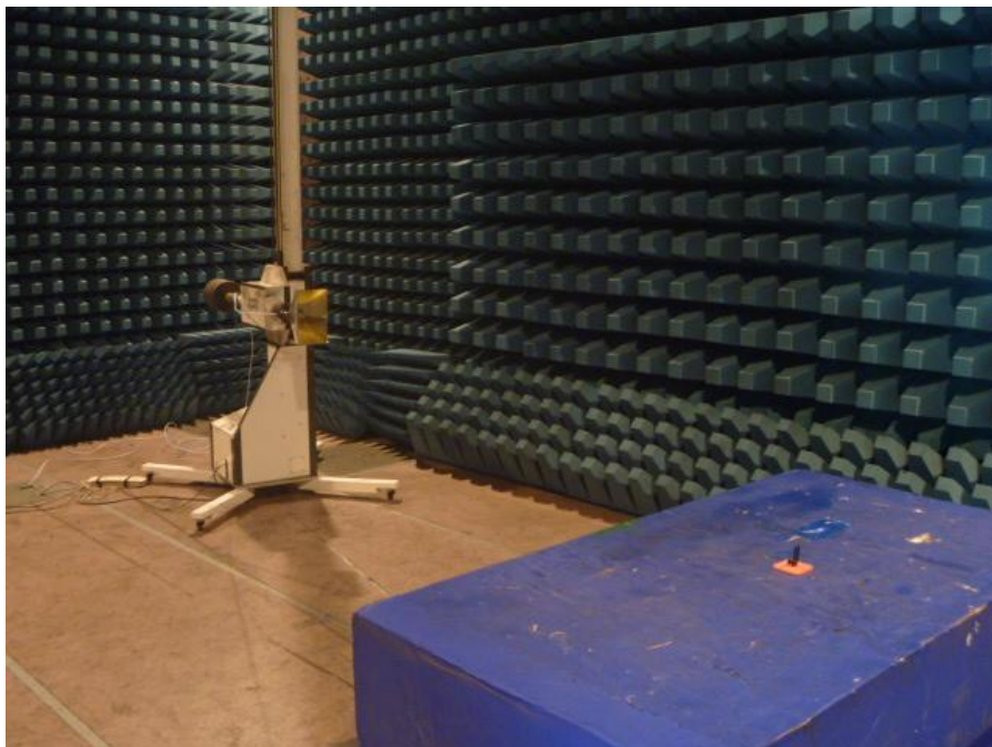
Z axis
