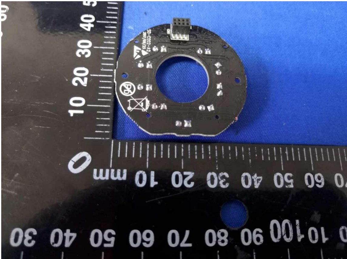
LED-Rear View(SVC563)
