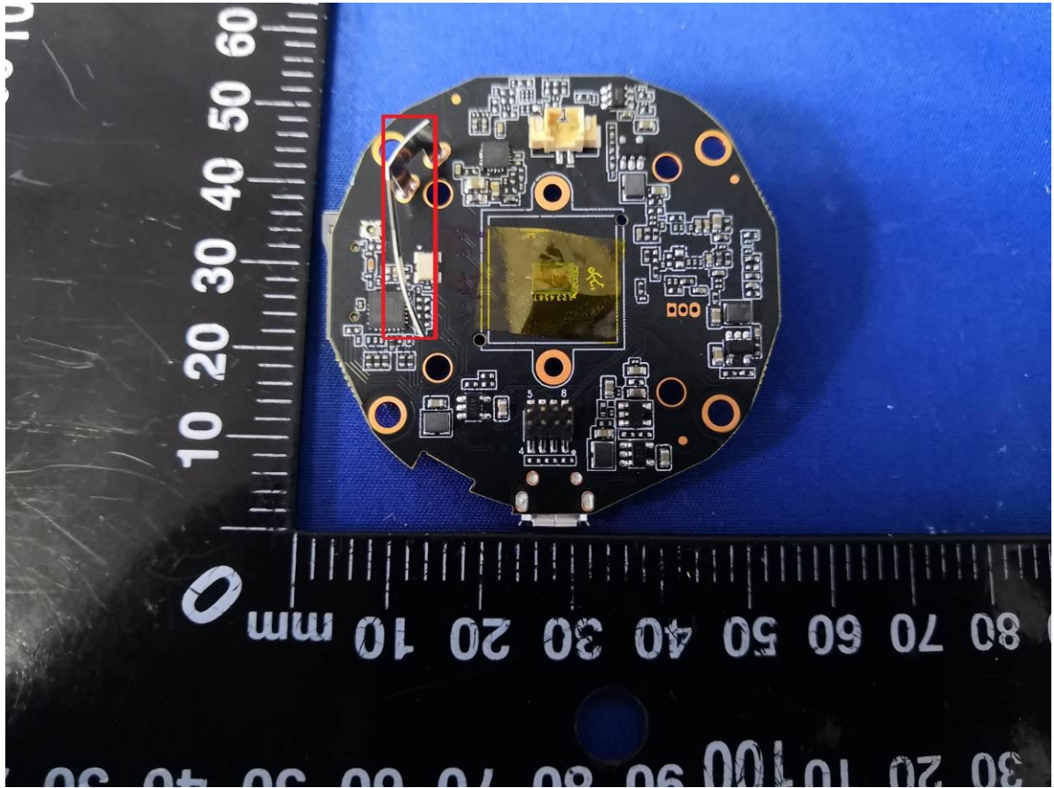
Antenna View(SVC562)
