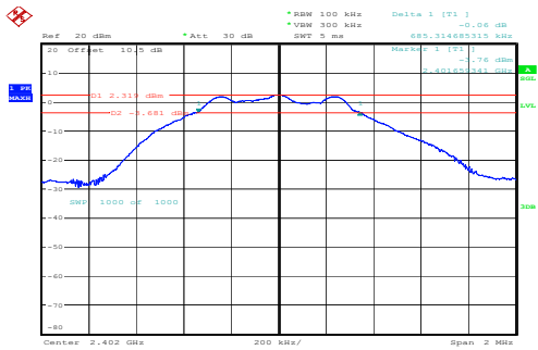
Low 0.685MHz
