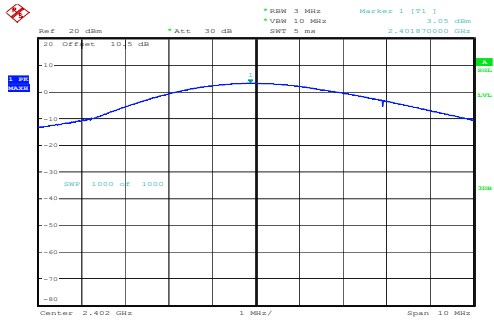
Low 3.05dBm
