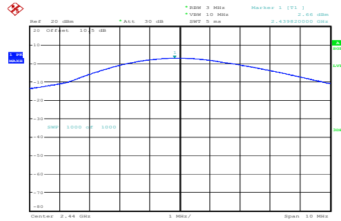
Middle 2.66dBm
