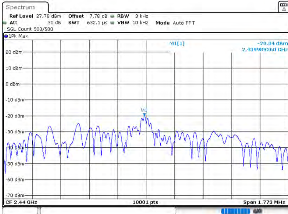
PSD NVNT BLE 2440MHz Ant0
