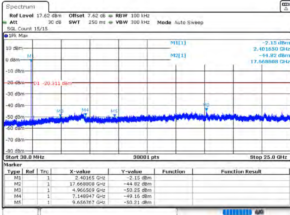
Tx. Spurious NVNT BLE 2402MHz Ant0 Emission
