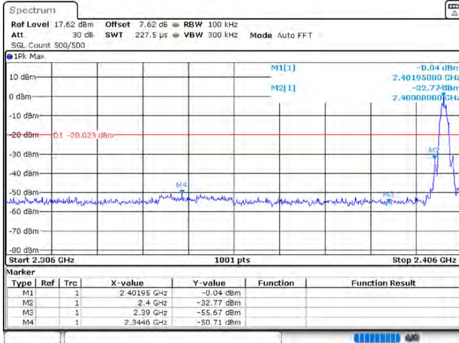
Band Edge NVNT BLE 2402MHz Ant0 Emission
