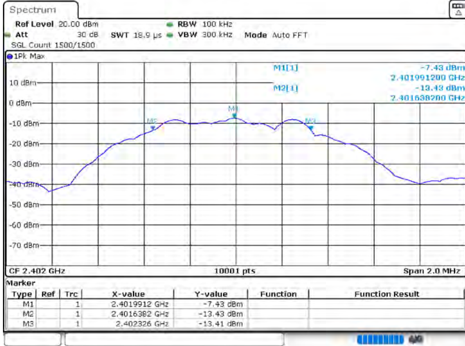
-6 dB BW NVNT BLE 2402MHz Ant0
