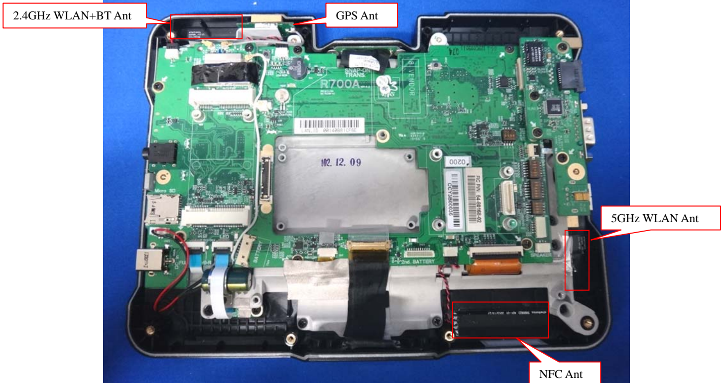
(16) EUT Photo
