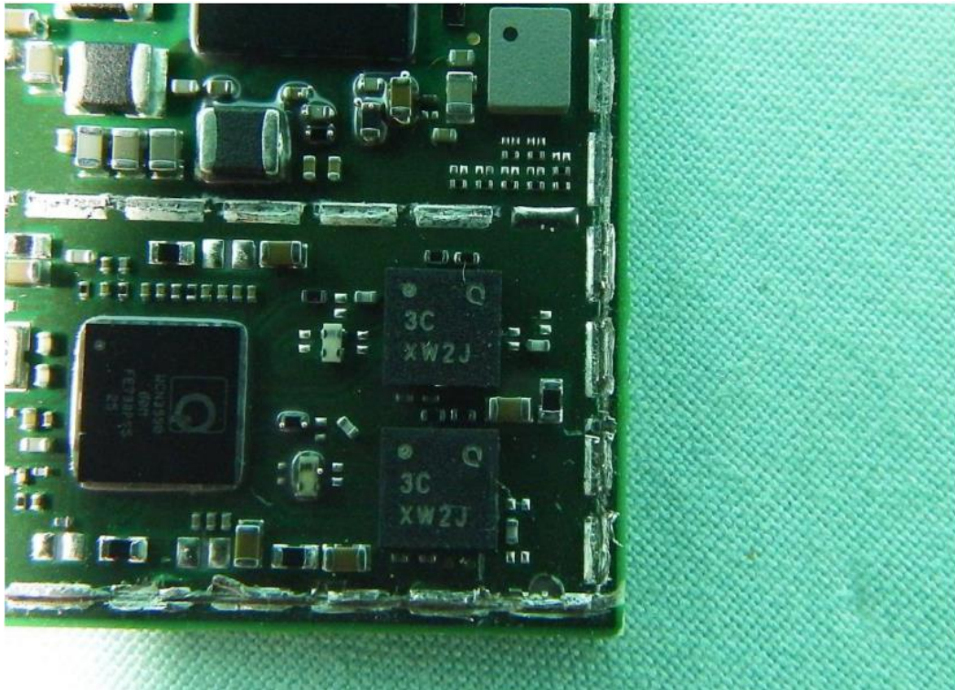
(15) EUT Photo
