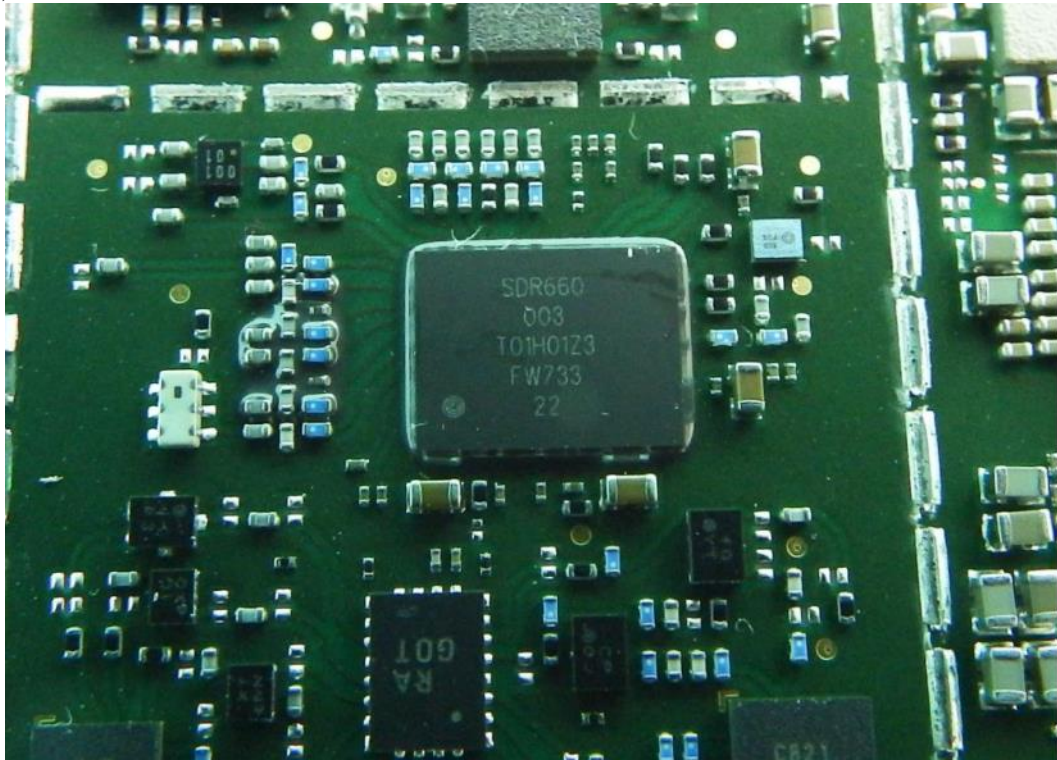
(9) EUT Photo
