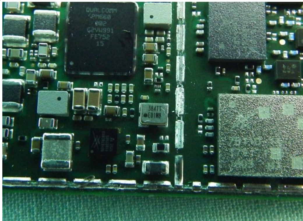
(8) EUT Photo
