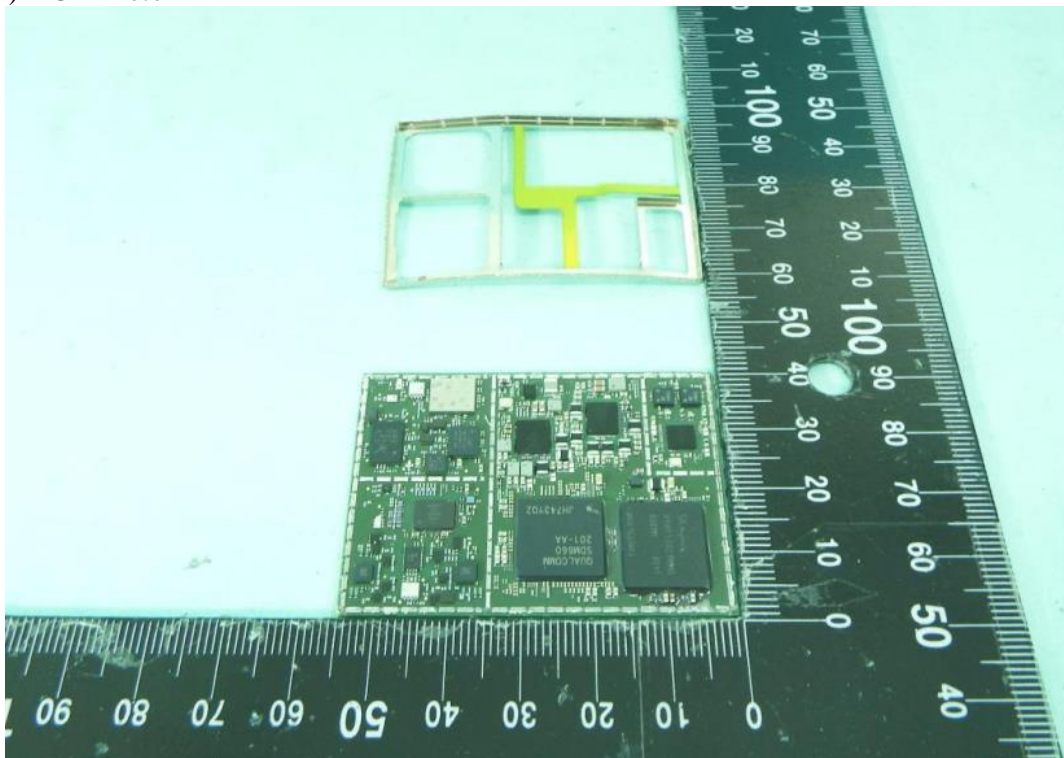
(2) EUT Photo
