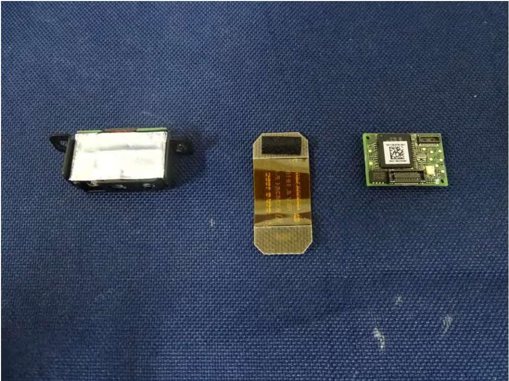
(46) EUT Photo
