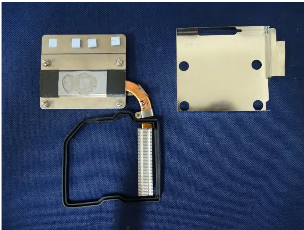
(41) EUT Photo
