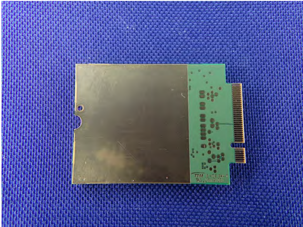
(65) EUT Photo
