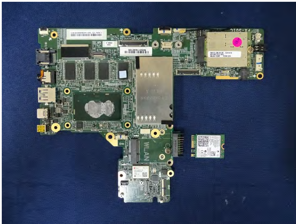
(57) EUT Photo
