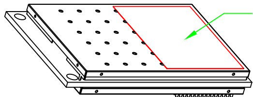
SA9800-A1 立體視圖
