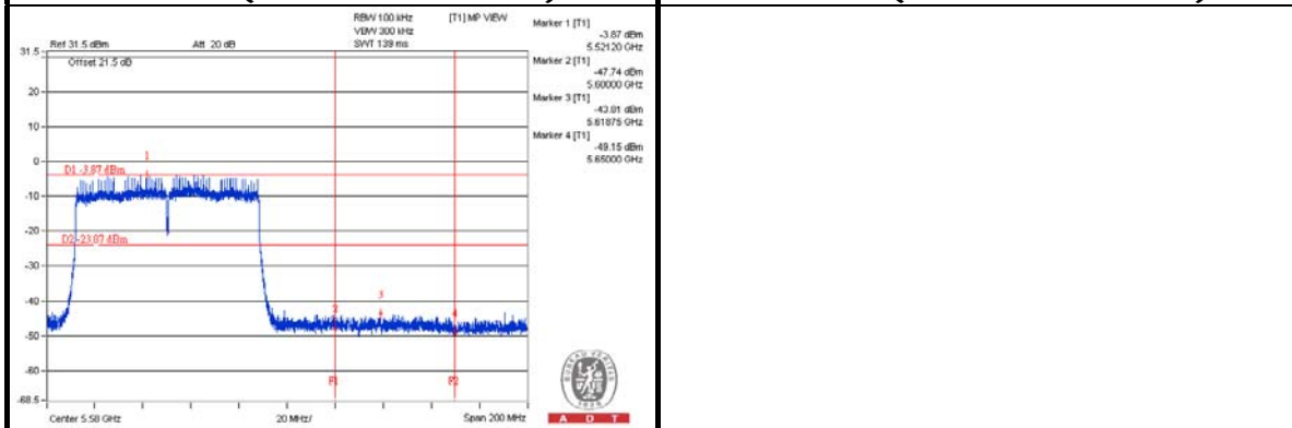
802.11ac (VHT 80MHz) OFDM MODULATION(CH 106: 5530MHz)
