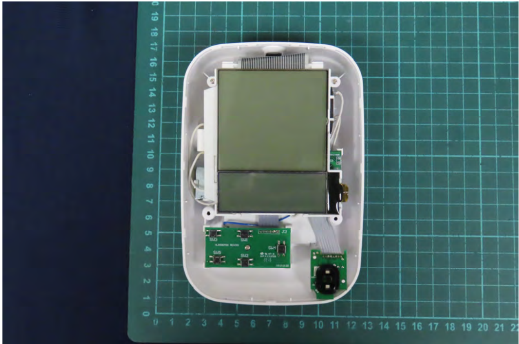
(3) EUT Photo
