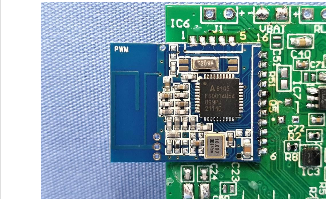
EUT Photo (6)
