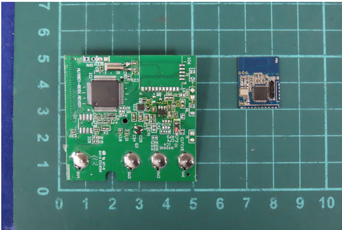
(9) EUT Photo
