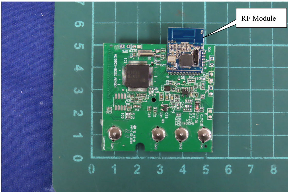
(8) EUT Photo
