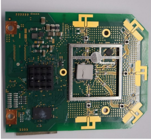
Q1025 – top side open shielding
