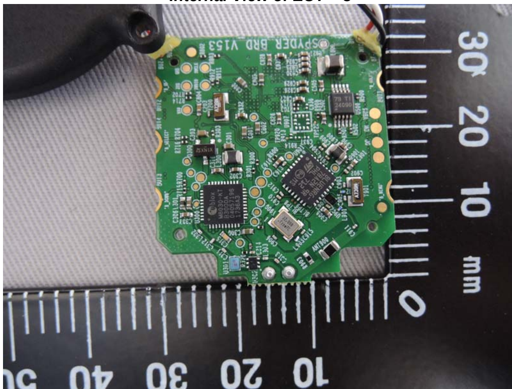
BLE Antenna
