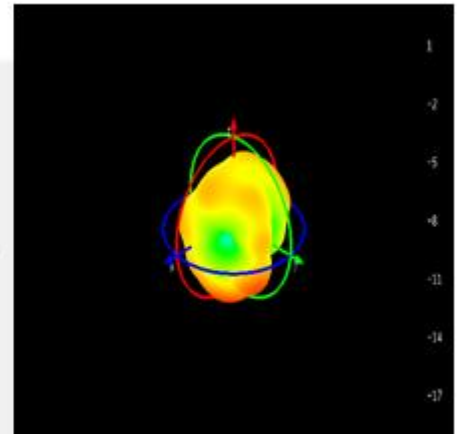
Theta=90 freq=1600MHz
