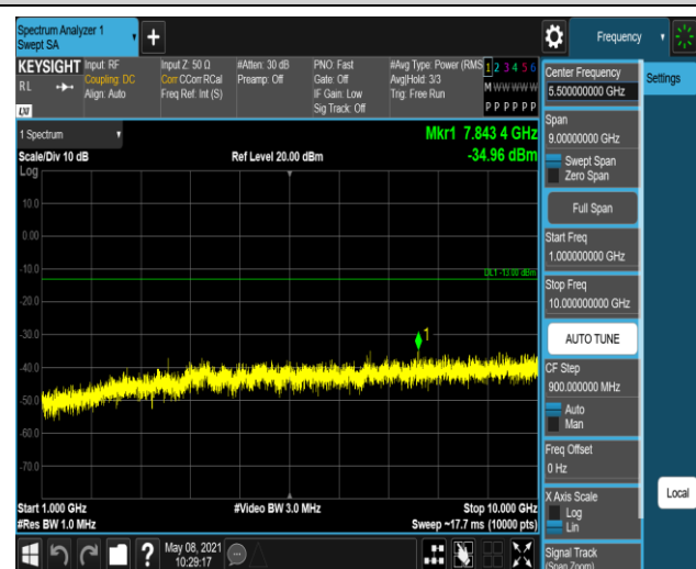
Band5-1.4MHz-QPSK-20525:1000~10000MHz
