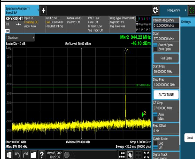
Band5-1.4MHz-QPSK-20525:30~1000MHz
