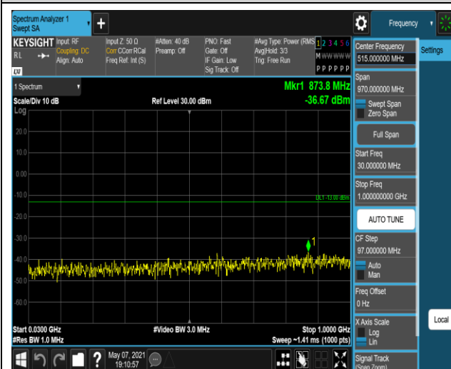
Band4-1.4MHz-QPSK-20393:30~1000MHz
