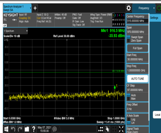
Band2-1.4MHz-QPSK-19193:30~1000MHz
