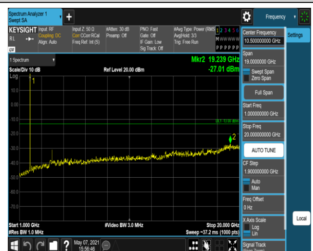
Band2-1.4MHz-QPSK-19193:1000~20000MHz
