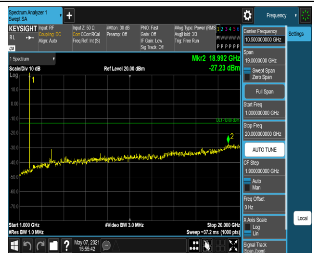
Band2-1.4MHz-QPSK-19193:1000~20000MHz
