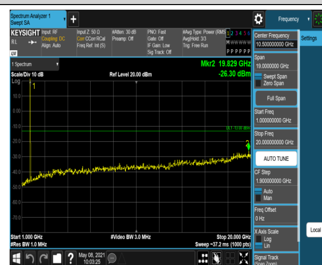
Band4-20MHz-QPSK-20175:1000~20000MHz
