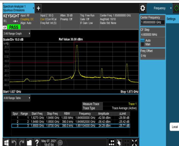
Band2-20MHz-QPSK-18700-100RB#0
