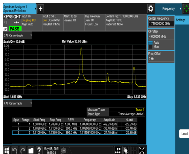
Band4-20MHz-QPSK-20050-100RB#0
