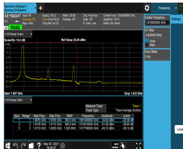
Band2-20MHz-QPSK-19100-100RB#0
