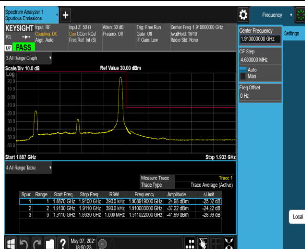
Band2-20MHz-QPSK-19100-1RB#99
