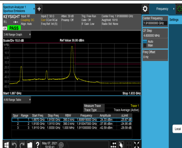
Band2-20MHz-16QAM-19100-1RB#99
