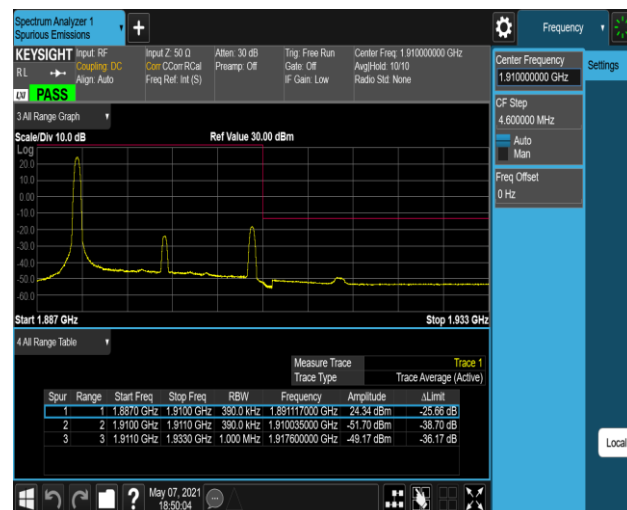
Band2-20MHz-16QAM-19100-100RB#0
