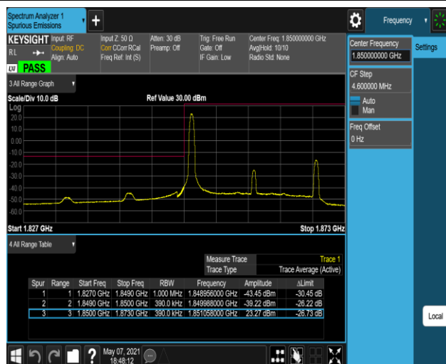
Band2-20MHz-16QAM-18700-100RB#0
