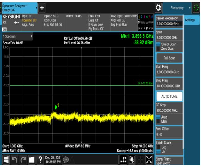
Band12-1.4MHz-QPSK-23017-1RB#0-Range2:1000~10000MHz
