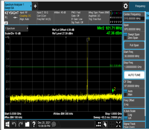
Band12-1.4MHz-QPSK-23017-1RB#0-Range1:30~1000MHz
