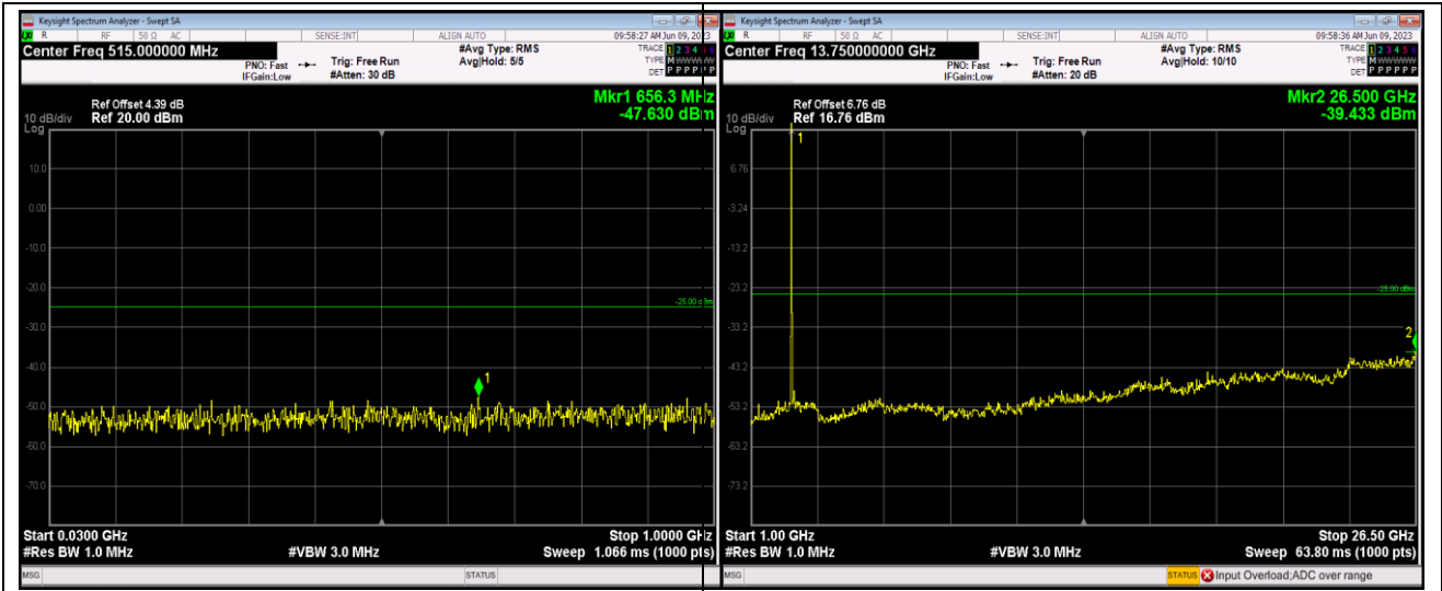
Band41-20MHz-16QAM-40740-1RB#0-Range1:30 ~1000MHz
