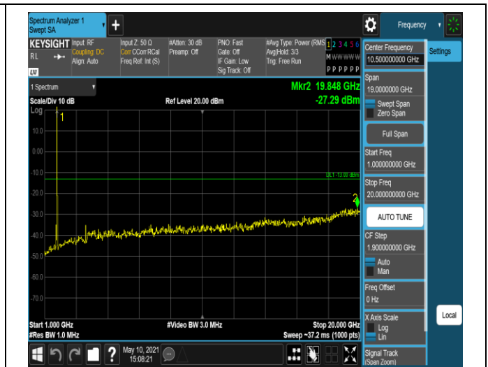
Band66-20MHz-QPSK-132572-1RB#0-Range2:1000~20000MHz
