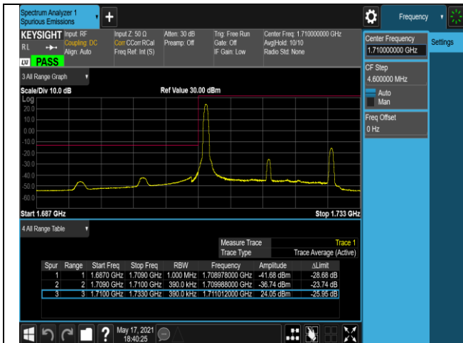
Band4-20MHz-QPSK-20050-100RB#0
