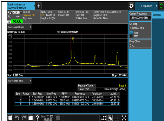
Band2-20MHz-QPSK-18700-100RB#0
