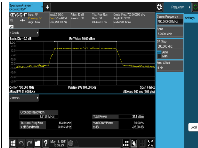
Band12-3MHz-QPSK-23165-15RB#0
