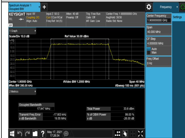
Band2-20MHz-16QAM-18900-100RB#0
