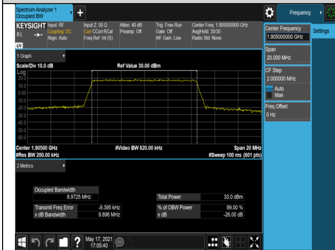
Band2-10MHz-16QAM-18900-50RB#0
