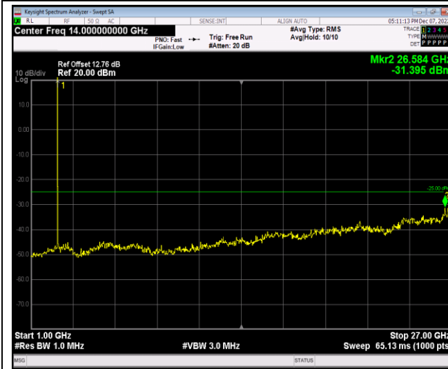
Band41-5MHz-16QAM-400265-1RB#0-Range2:1000~27000MHz
