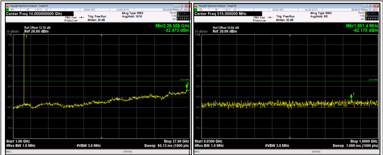
Band41-5MHz-16QAM-41215-1RB#0-Range2:1000~27000MHz
