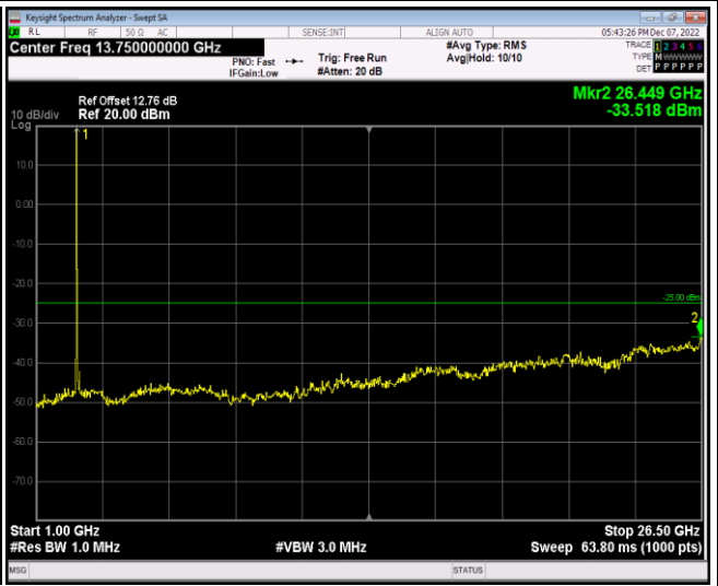
Band41-20MHz-QPSK-40340-1RB#0-Range2:1000~26500MHz
