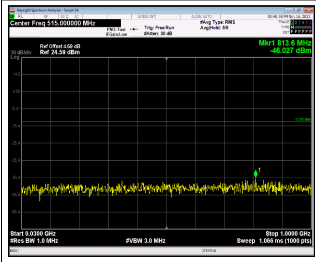
Band2-20MHz-16QAM-18700-1RB#0-Range1:30~10 00MHz
