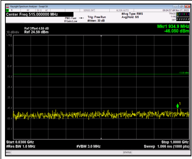
Band4-1.4MHz-QPSK-20393-1RB#0-Range1:30~1000MHz
