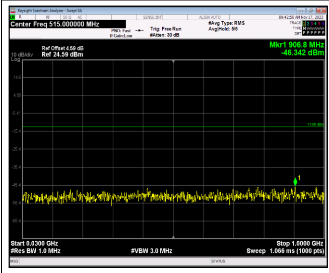
Band4-20MHz-QPSK-20175-1RB#0-Range1:30~100 OMHz
