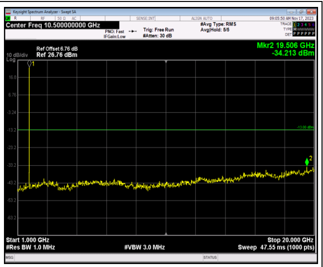
Band4-20MHz-QPSK-20050-1RB#0-Range2:1000~20000MHz
