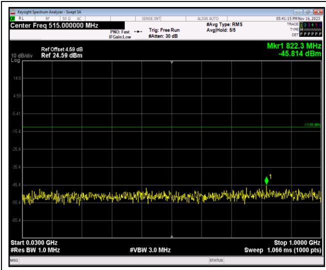
Band2-20MHz-QPSK-19100-1RB#0-Range1:30~100 0MHz
