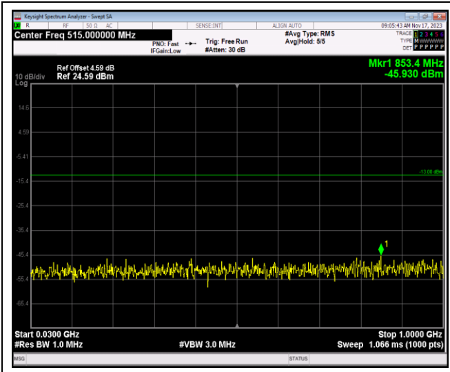
Band4-20MHz-QPSK-20050-1RB#0-Range1:30~100 OMHz
