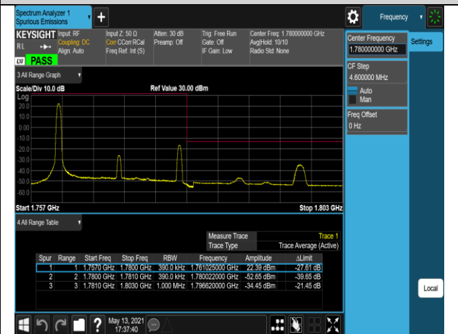
Band66-20MHz-QPSK-132572-100RB#0
