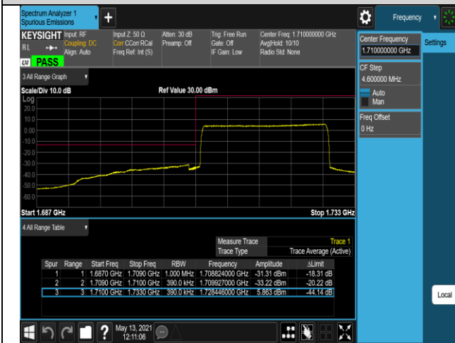
Band4-20MHz-QPSK-20300-1RB#99
