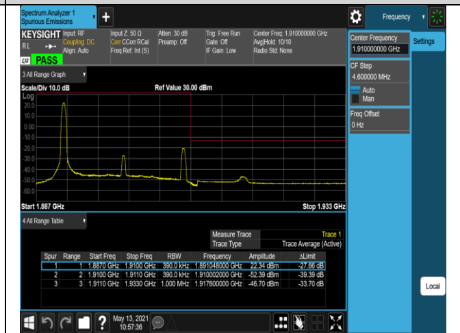
Band2-20MHz-16QAM-19100-100RB#0
