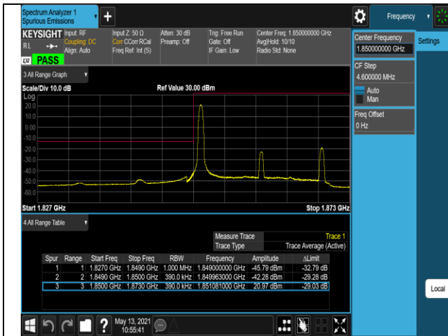
Band2-20MHz-16QAM-18700-100RB#0
