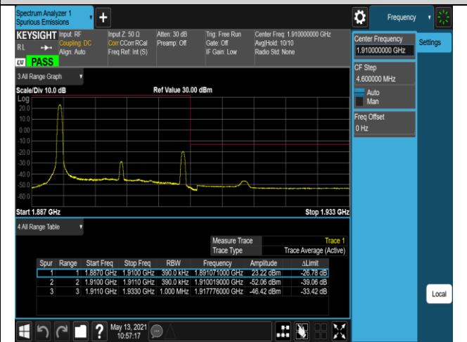
Band2-20MHz-QPSK-19100-100RB#0
