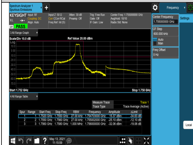
Band4-20MHz-QPSK-20050-1RB#0
