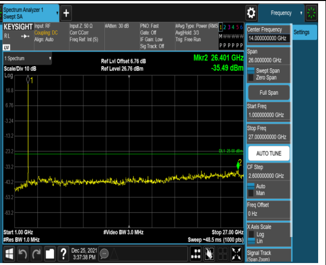
Band7-20MHz-QPSK-21350-1RB#0-Range2:1000~27000MHz
