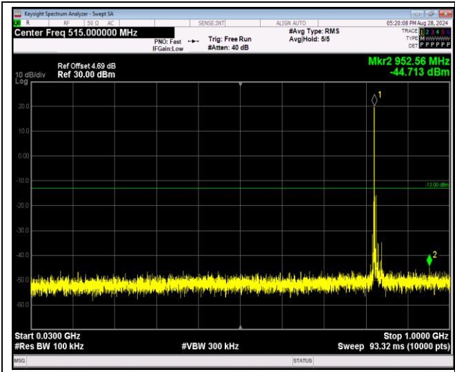
Band5-10MHz-QPSK-20525-1RB#0-Range1:30~100 OMHz
