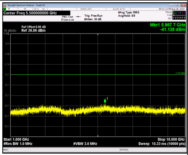
Band5-10MHz-QPSK-20600-1RB#0-Range2:1000~1 0000MHz
