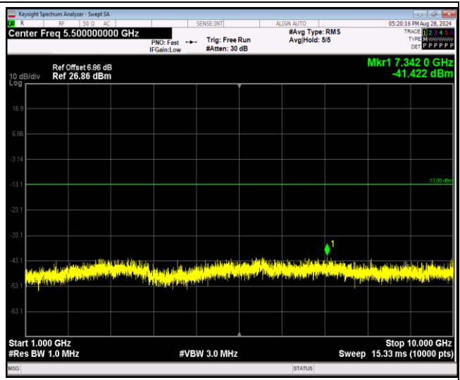
Band5-10MHz-QPSK-20525-1RB#0-Range2:1000~1 0000MHz
