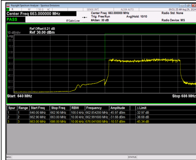
Band71-20MHz-64QAM-133372-1RB#99
