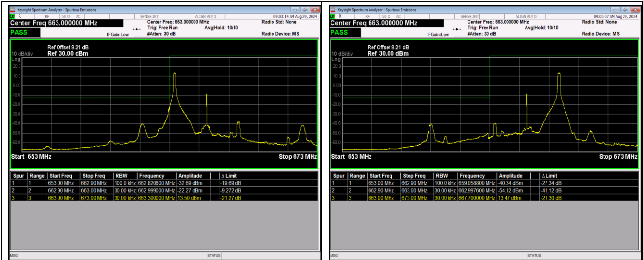
Band71-5MHz-QPSK-133147-25RB#0
