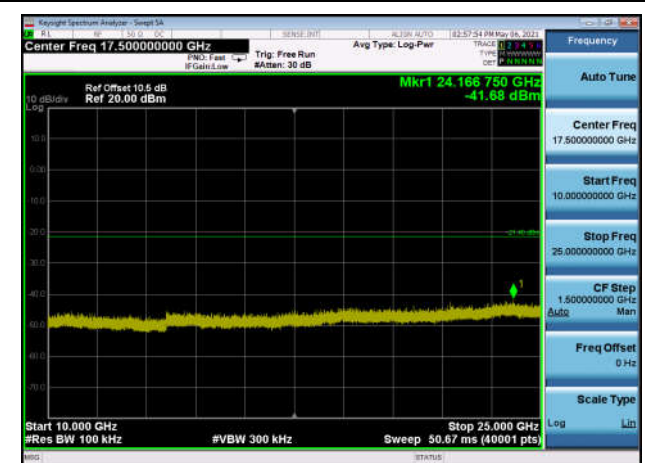
,Plot 5,10000MHz~25000MHz-802.11n(HT40),2452MHz,Ant0
