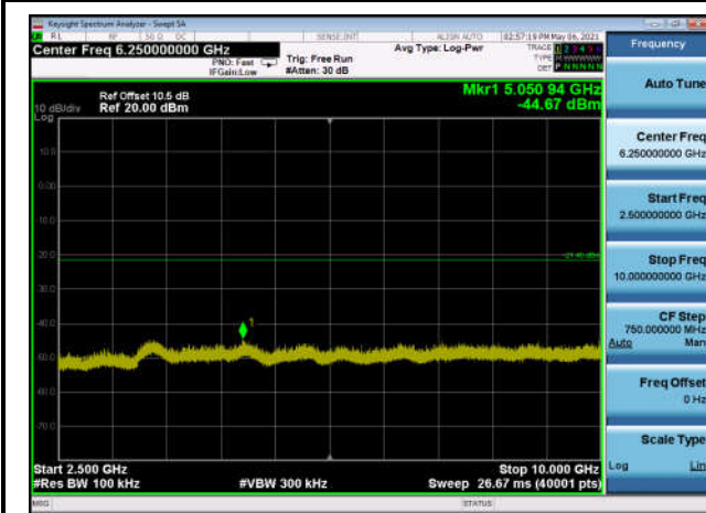
,Plot 4,2500MHz~10000MHz-802.11n(HT40),2452MHz,Ant0
