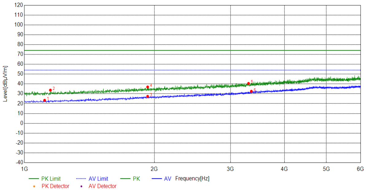
(Plot A: Test Antenna Horizontal 1G – 6G)
