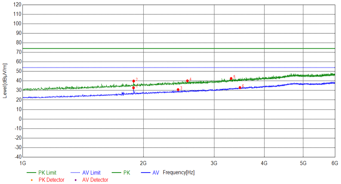
(Plot A: Test Antenna Horizontal 1G – 6G)
