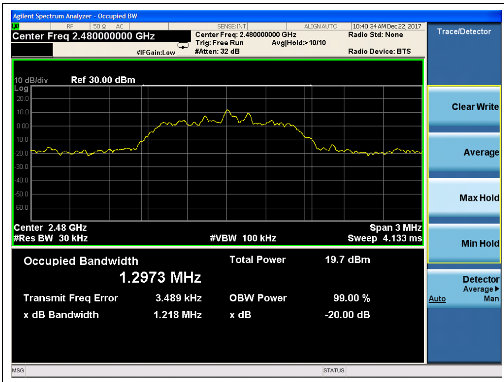
( \pi/4 -DQPSK, Channel 39, 2480MHz)
