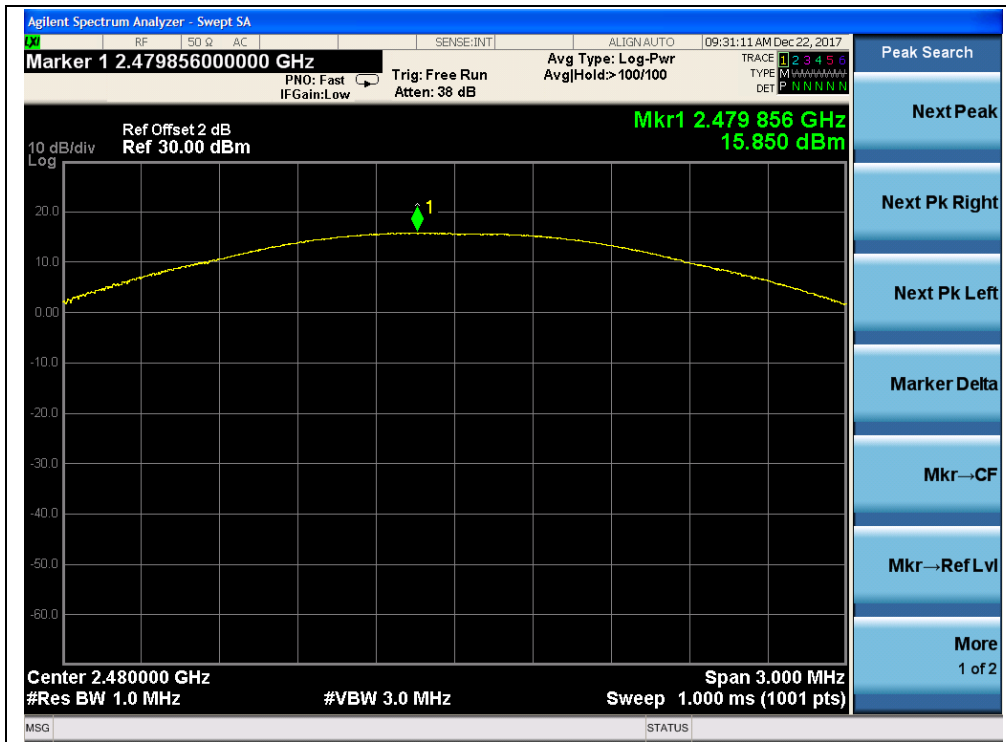
( \pi/4 -DQPSK, Channel 39, 2480MHz)
