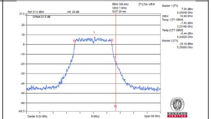
802.11a_Chain 3 / CH48
