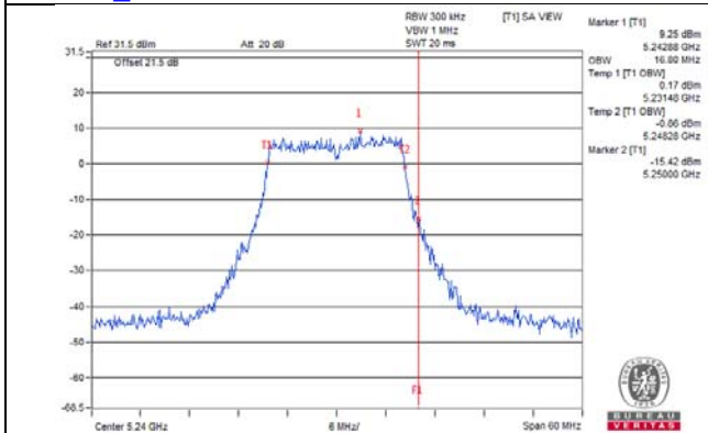
802.11a_Chain 4 / CH48
