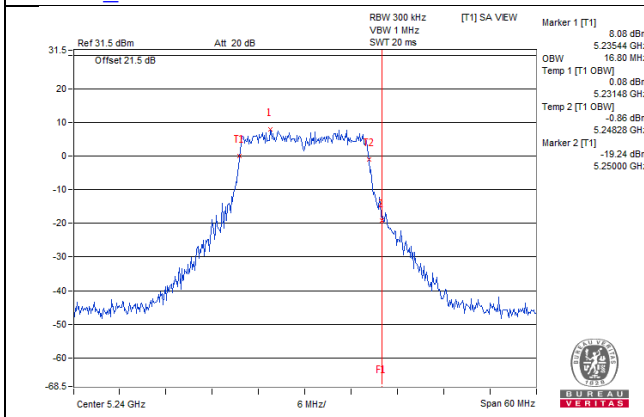
802.11a_Chain 6 / CH48
