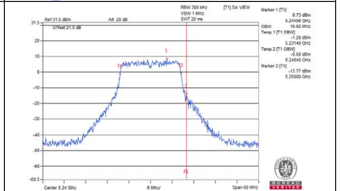
802.11a_Chain 7 / CH48
