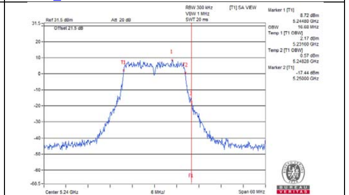
802.11a_Chain 5 / CH48
