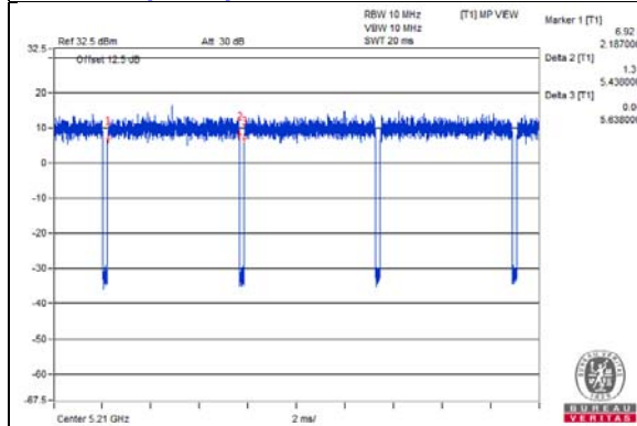
802.11ax (HE80)
