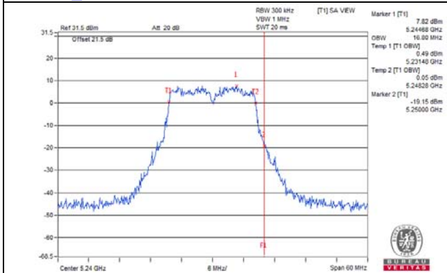
802.11a_Chain 6 / CH48
