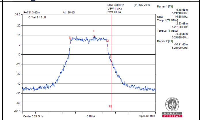
802.11a_Chain 7 / CH48
