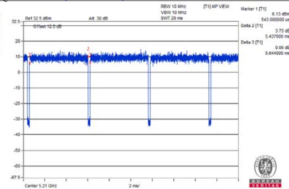
802.11ax (HE80+80)
