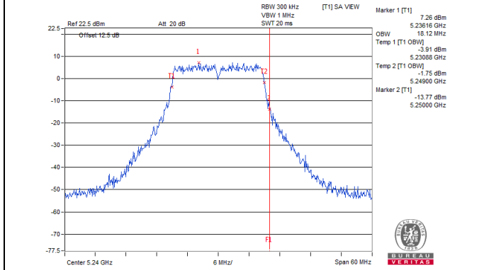
802.11ac (VHT20)_Chain 2 / CH48
