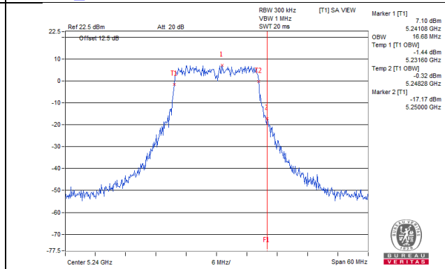
802.11a_Chain 7 / CH48
