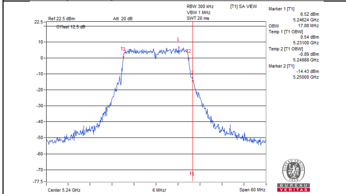
802.11ac (VHT20)_Chain 6 / CH48
