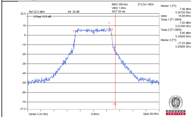
802.11a_Chain 6 / CH48
