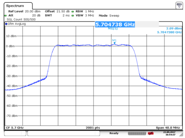
Channel 140 (5700MHz)
