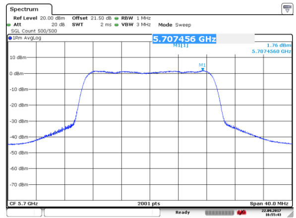
Channel 140 (5700MHz)
