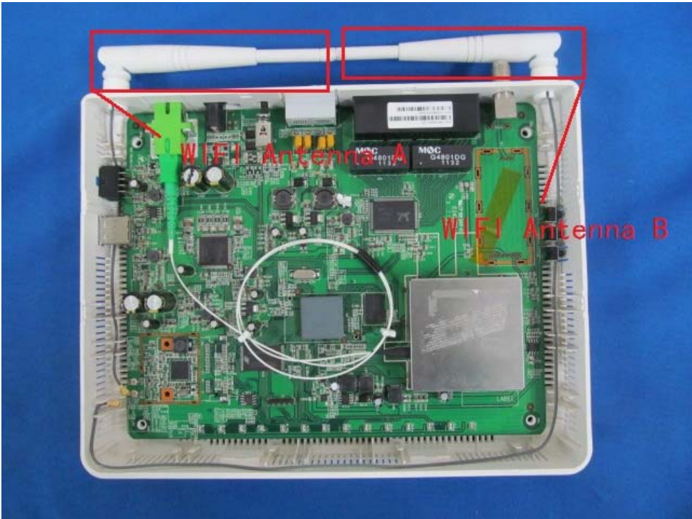
(2) EUT Photo (TO77G)
