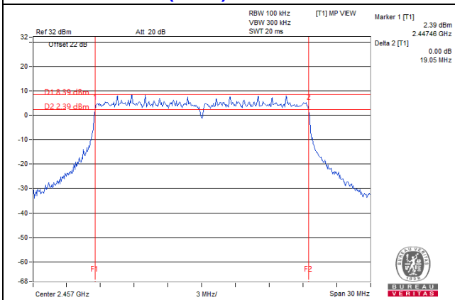
802.11ax (HE20) / Chain 1 : CH10
