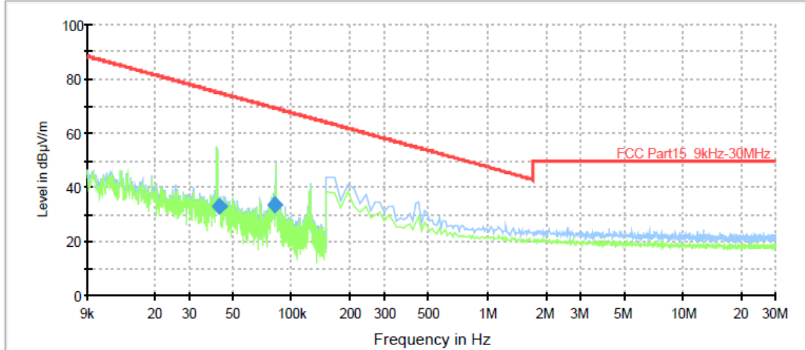
RE 9K-30MHz
