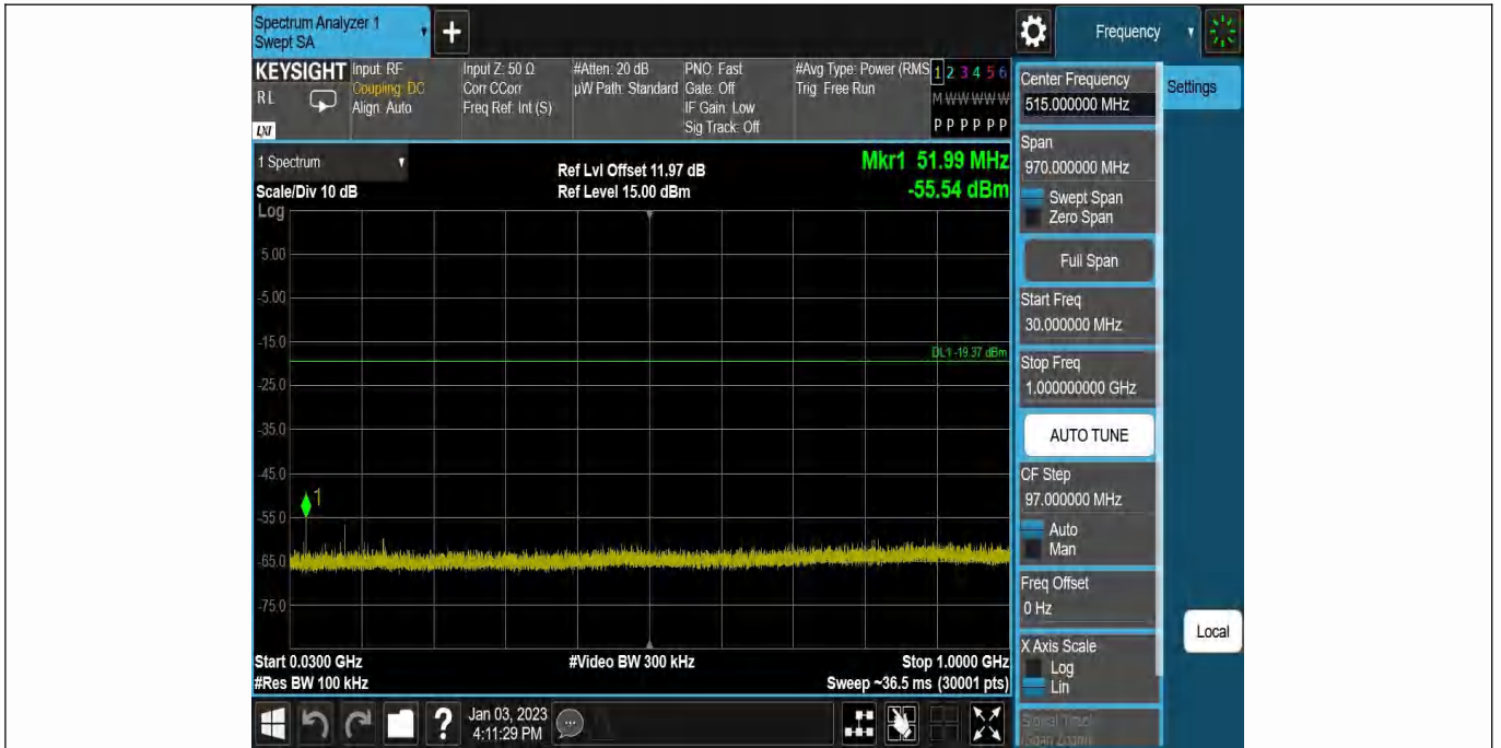
DH5-Ant1-2441-30~1000-0.63
