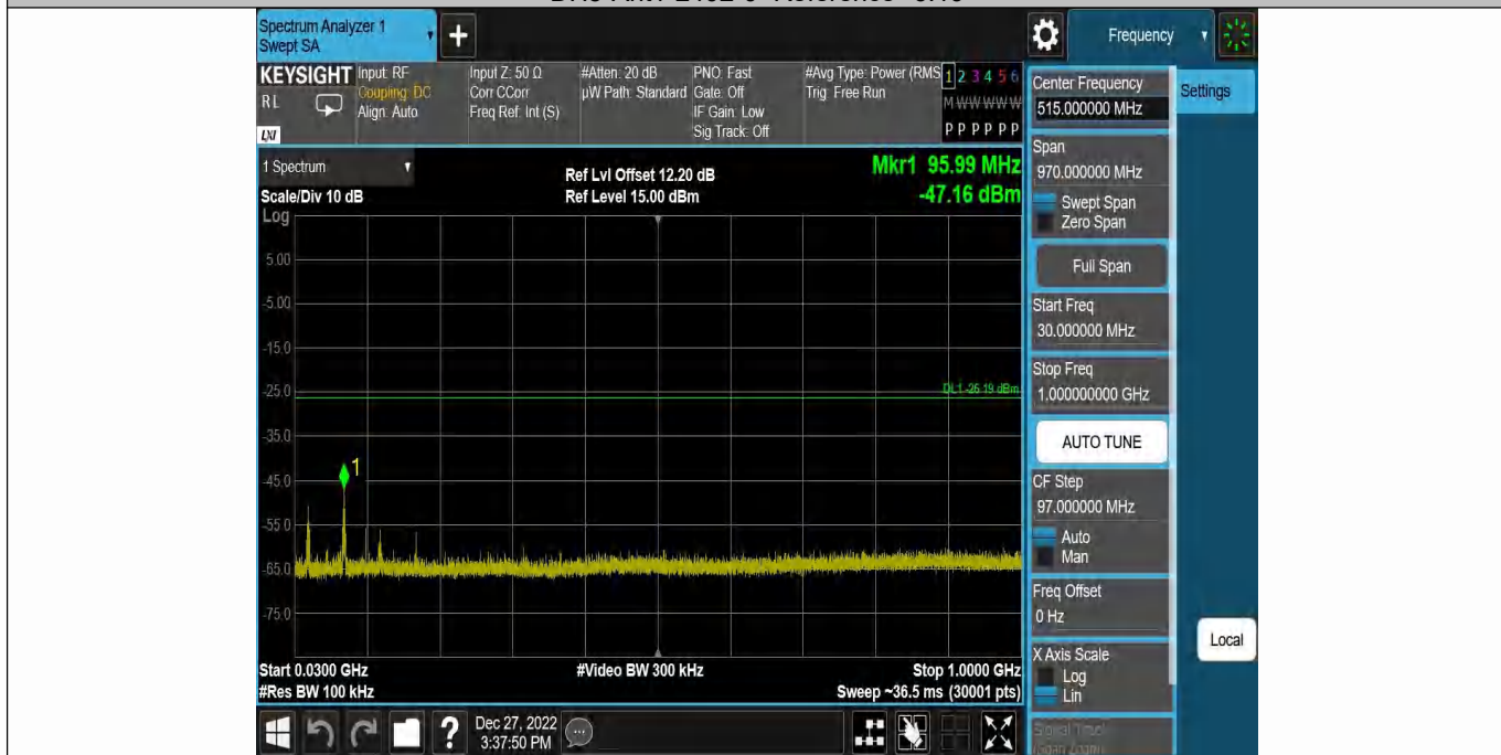
DH5-Ant1-2402-30~1000--6.19
