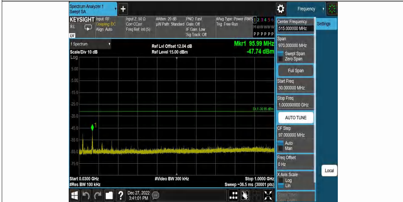
DH5-Ant1-2480-30~1000--10.95
