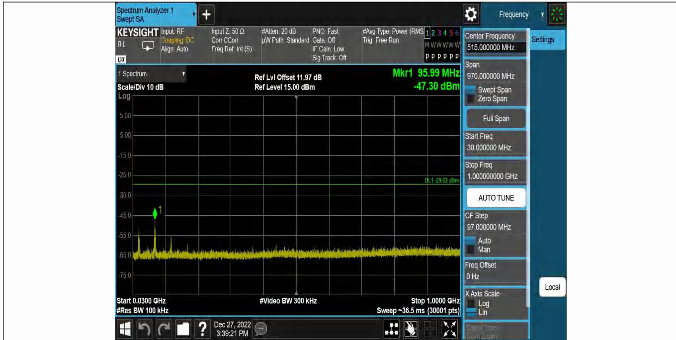
DH5-Ant1-2441-30~1000--9.63
