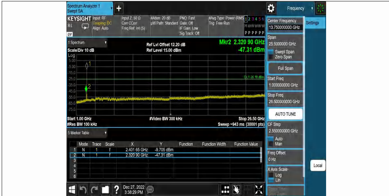
DH5-Ant1-2402-1000~26500~-6.19
