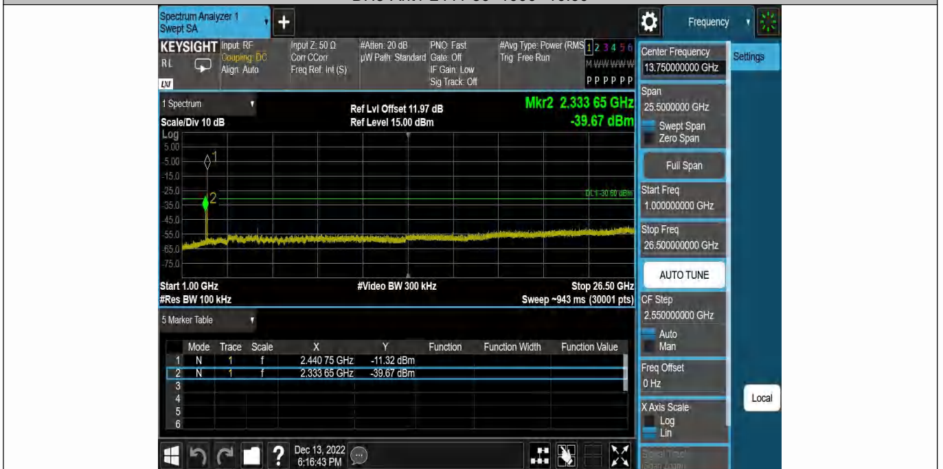
DH5-Ant1-2441-1000~26500--10.60
