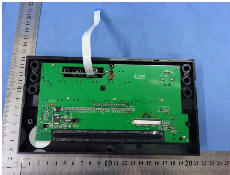
KEY&DISPLAR BOARD
