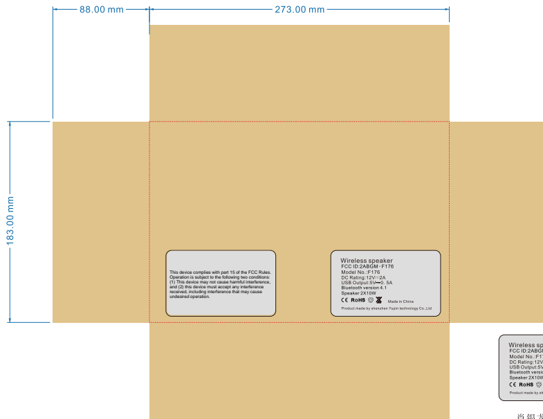
地盒（折好外尺寸：长273*宽183*高88）
