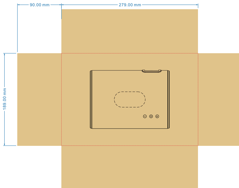
天盒（折好外尺寸：长279*宽189*高90）
