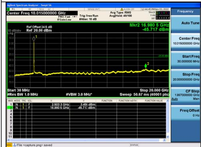
Band41C-30M-20G / 20MHz+15MHz / 100RB+75RB/ QPSK / LOW CH
