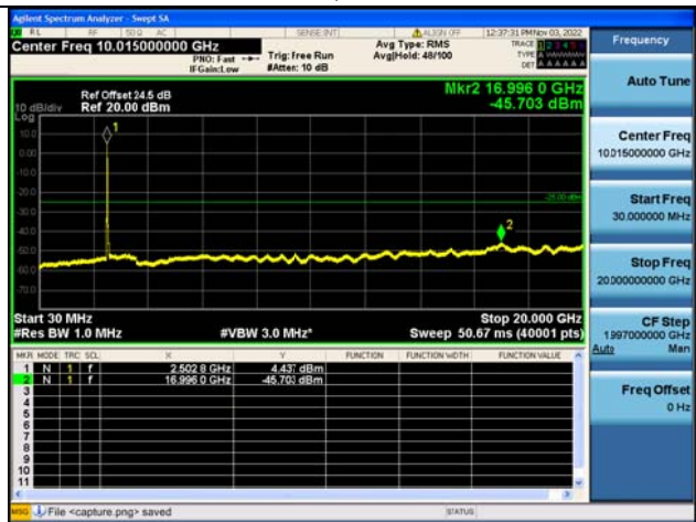
Band41C-30M-20G / 10MHz+20MHz / 50RB+100RB/ QPSK / LOW CH
