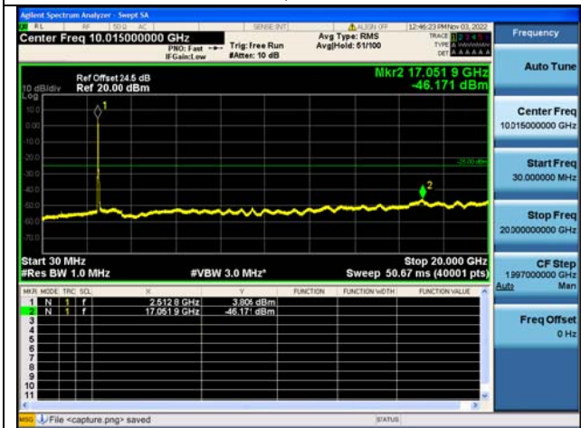
Band41C-30M-20G / 20MHz+20MHz / 100RB+100RB/ QPSK / LOW CH
