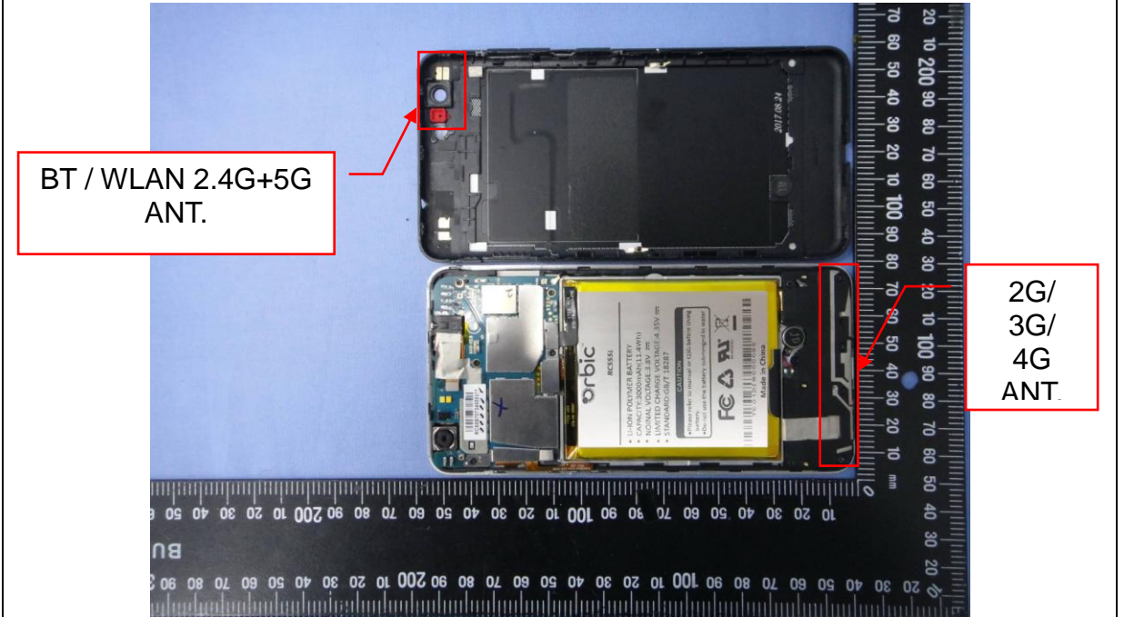
EUT Photo (2)
