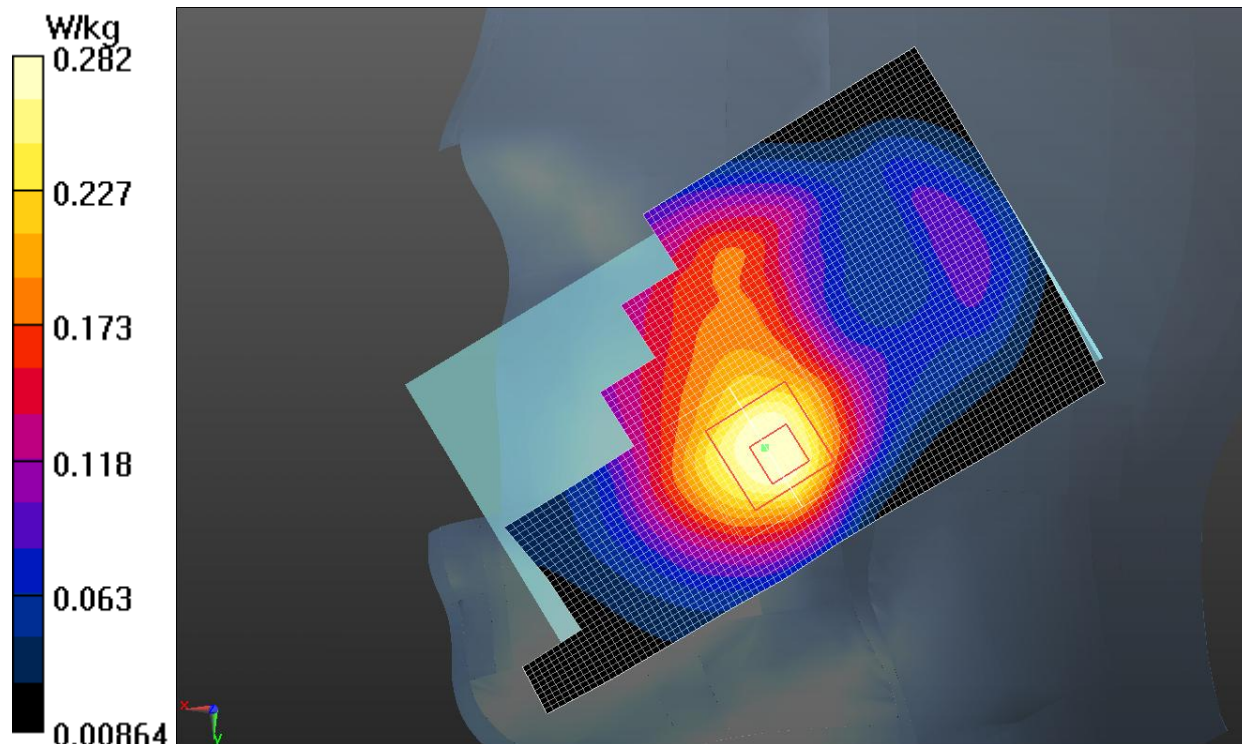
Fig.9 WCDMA1700 CH1413
